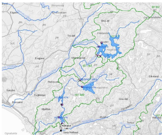
Figur, Hetland kraftverk med tilhørende vannmagasiner.
